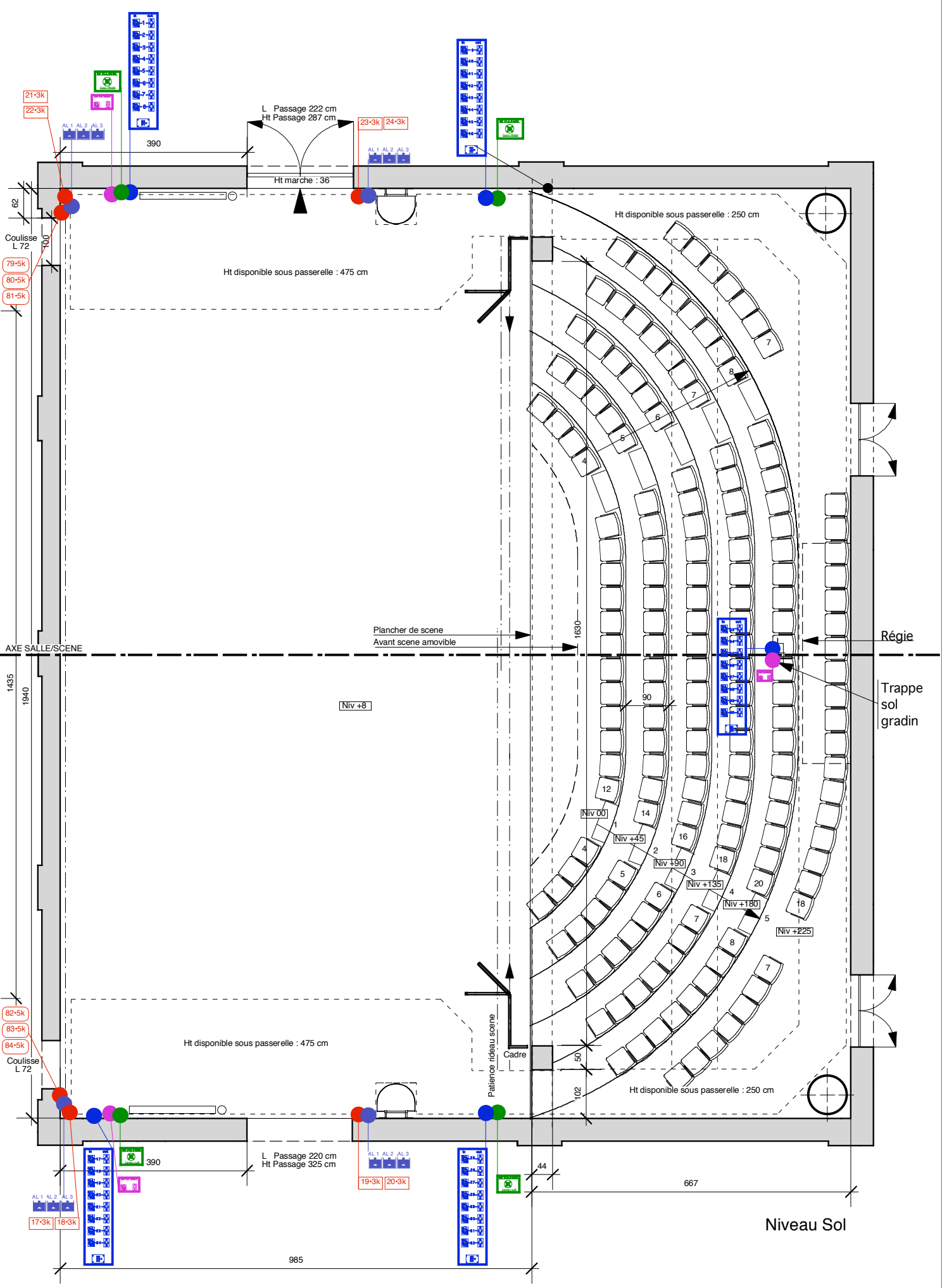
THEATRE DE LA BALSAMINE av Félix Marchal 1 à 1030 Bruxelles GRANDE SALLE échelle : 1cm par m
